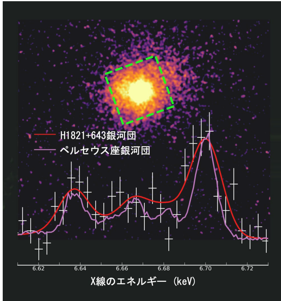
図 2. チャンドラ X 線天文衛星による H1821+643 銀河団の X 線画像。緑の点線は、1 辺約 90 万光年の観測領域を示す。下図は中心領域（半径約 30 万光年）における鉄イオン（6.7 keV（キロ電子ボルト）など）の X 線輝線のエネルギー分布で、観測データ（白）とモデル（赤）を重ねている。代表的な銀河団（ペルセウス座銀河団、紫）と比べ、線幅の広がりは顕著であり、広範囲で高温ガスの運動が激しいことがわかる。（クレジット：Yamada et al.）
