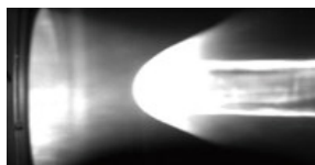
極超音速風洞ではやぶさ模型
