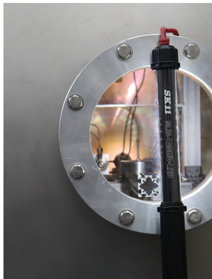
旋回型ハイブリッドロケットエンジンの燃焼実験
