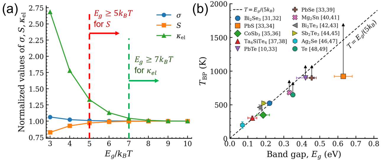
図 1. (a) バンドギャップ E_g を変化させたときのゼーベック係数 S と電子熱伝導率 \kappa_{el} の変化。一般に、バンドギャップ E_g が大きいほどバイポーラ効果は生じにくくなる。 S については E_g \geq 5k_B T 、 \kappa_{el} については E_g \geq 7k_B T を満たせば、バイポーラ効果による |S| の減少を 5%以下、 \kappa_{el} の増加を 10%以下に抑えられることが分かる。(b) さまざまな熱電材料の最適組成における、バイポーラ効果が現れる温度 T_{BP} のバンドギャップ E_g 依存性。データはおおむね T_{BP} = E_g/(5k_B) の直線に沿う。なお、文献の測定温度範囲内でバイポーラ効果が確認されなかった物質は、測定範囲の最高温度にプロットし、矢印を付した。
