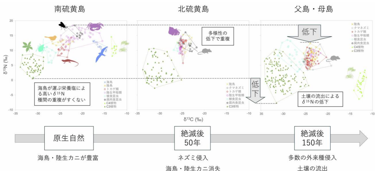
図2 南硫黄島、北硫黄島、父島・母島における窒素循環
